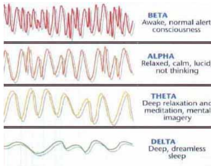
Die vier verschiedenen Hauptgehirnwellen
