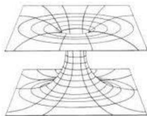
Eine Einstein-Rosen Brücke
